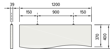
Modul 1200 x 400 mm
